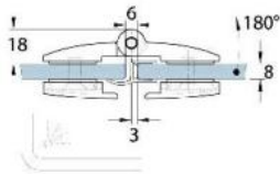
Mit Dichtprofil // with use of seal (Art.-Nr. // art.no. 69090)
