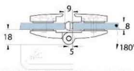
Glasbearbeitung // glass machining Mit Dichtprofil Art.-Nr. 69030 o. 69230 with use of seal art. nr. 69030 or 69230
