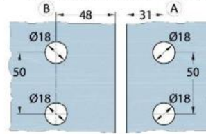
Mit Dichtprofil Art.-Nr. 69030 o. 69230 with use of seal art. nr. 69030 or 69230
