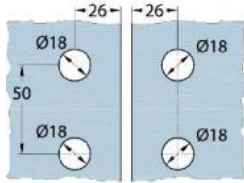
Mit Dichtprofil // with use of seal (Art.-Nr. // art.no. 69090)
