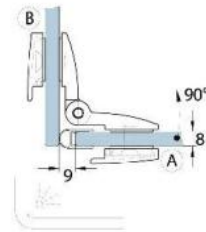
Mit Dichtprofil Art.-Nr. 69030 o. 69230 with use of seal art. nr. 69030 or 69230
