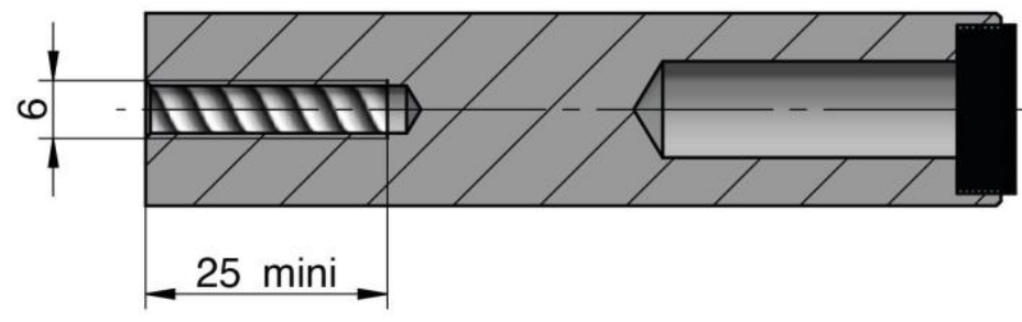
COUPE A-A
