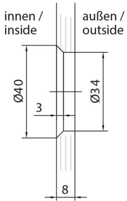
Fixteil / fixed panel
