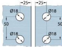
Mit Dichtprofil Art.-Nr. 69030 o. 69230 with use of seal art. nr. 69030 or 69230
