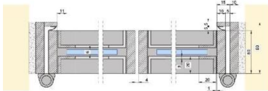
Höhenschnitt / coupe transversale
