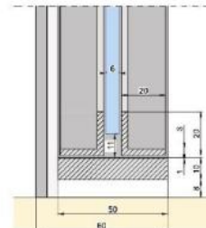
Seitenschnitt / coupe verticale
