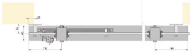
Höhenschnitt / coupe transversale
