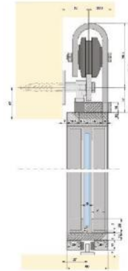
Seitenschnitt / coupe verticale
