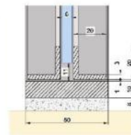
Seitenschnitt / coupe verticale
