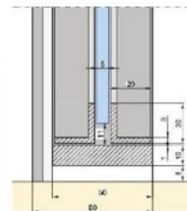
Seitenschnitt / coupe verticale
