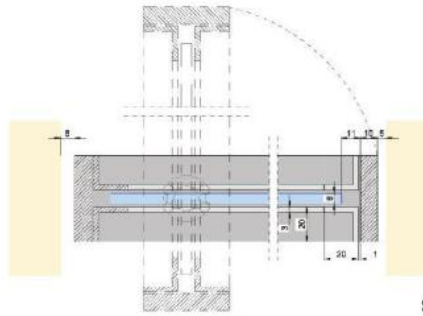
Höhenschnitt / coupe transversale
