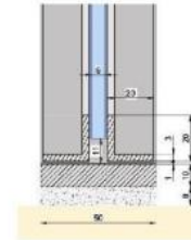
Seitenschnitt / coupe verticale
