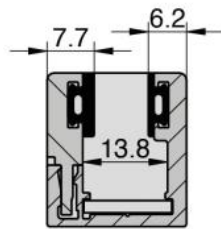
COUPE B-B
