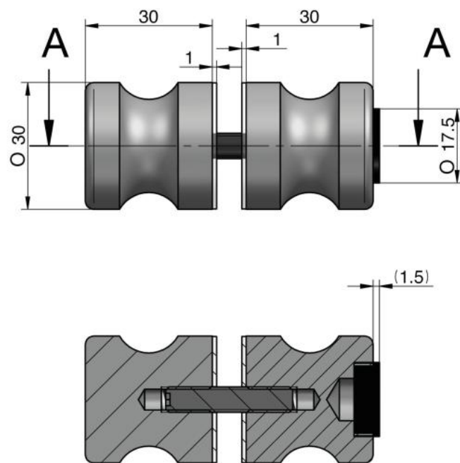
COUPE A-A
